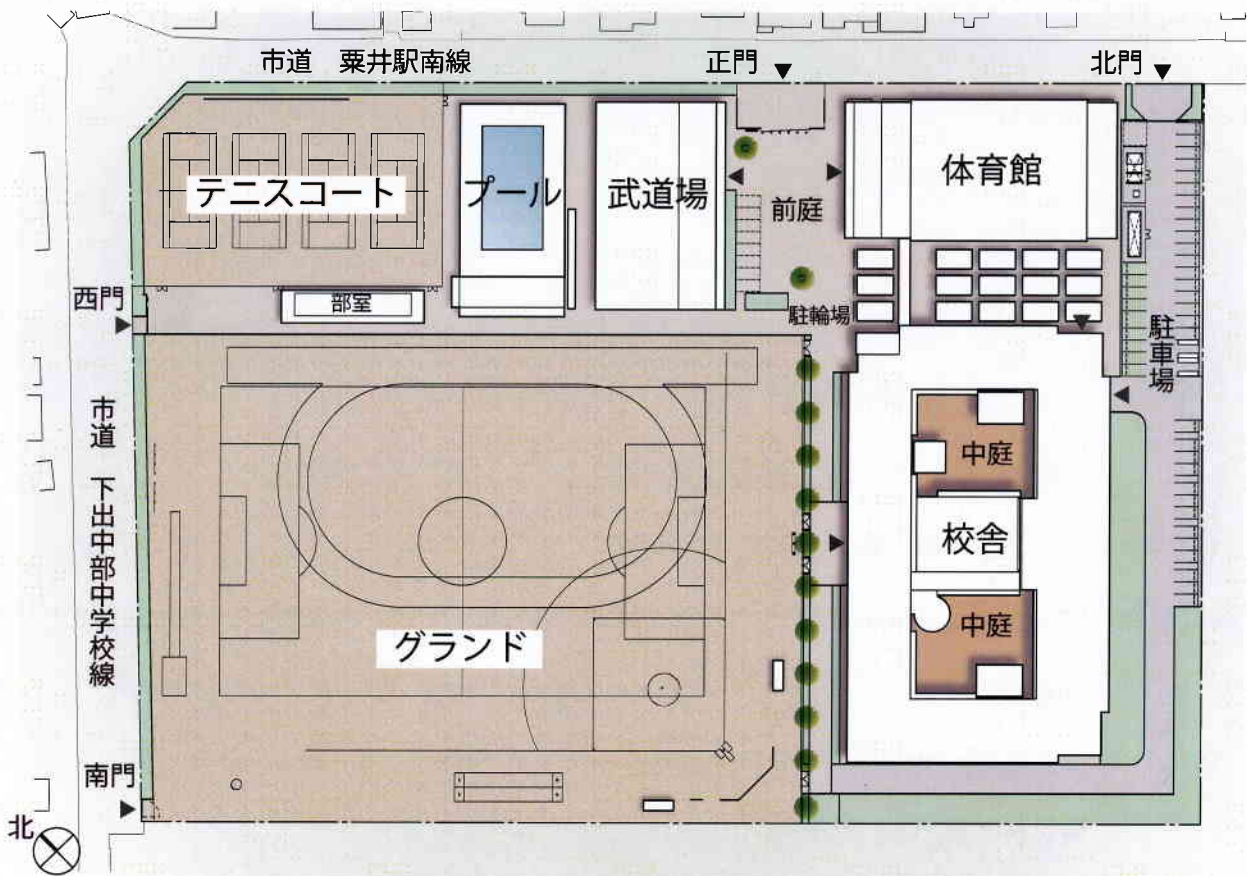
中部中学校 配置図
